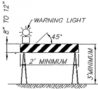
TYPE I BARRICADE
